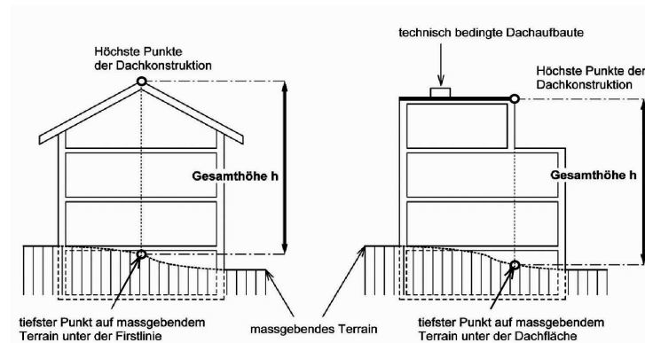
Figur 4.1.a Gesamthöhe
